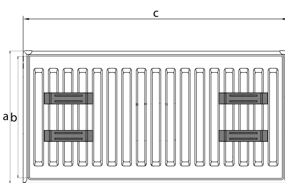
4 mensol için | 4 hangers ; 400/...../1700 mm
