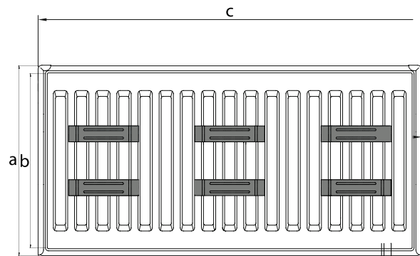
6 mensol için | 6 hangers; 1800/...../3000 mm
