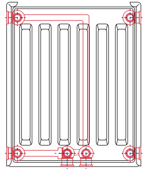
Ortadan Giriş Çıkışlı Middle Connection
