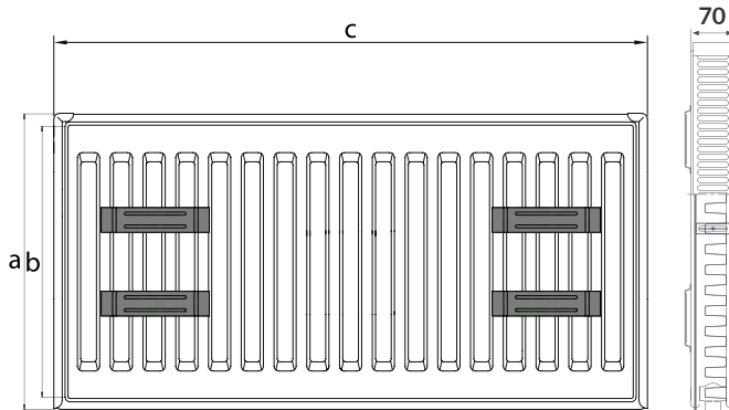
4 mensol için | 4 hangers ; 400/...../1700 mm
