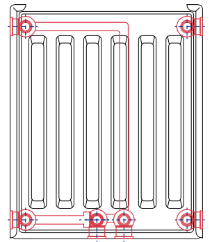
6 Giriş-Çıkışlı Ortadan Giriş Çıkışı 6 Holes Compac Middle Connection
