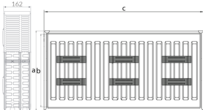
6 mensol için | 6 hangers; 1800/...../3000 mm
